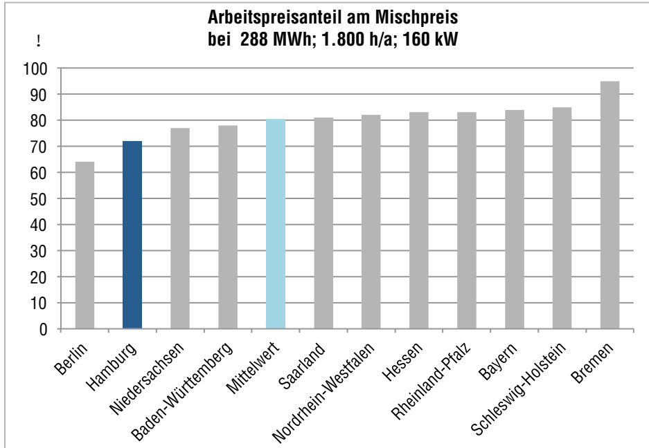
Abbildung 10: Arbeitspreisanteil am Mischpreis für Ausnutzungsdauer von 1.800 h/a und Anschlussleistung
