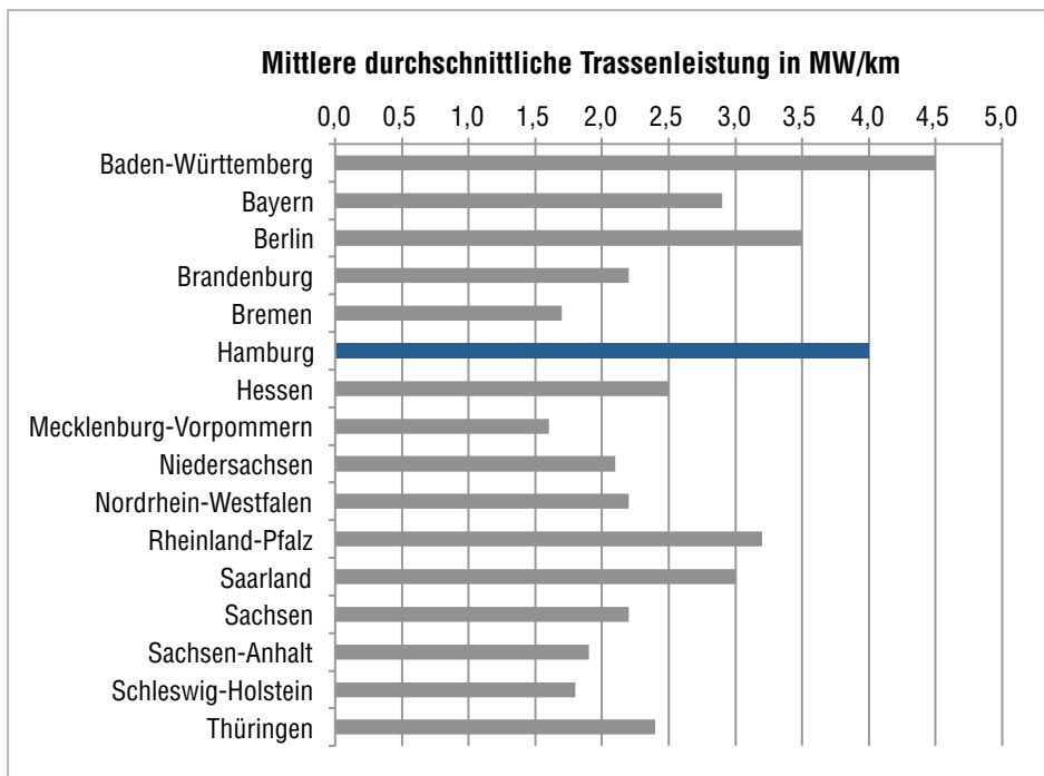
Abbildung 7: Mittlere Trassenleistung im Ländervergleich, Daten 45
