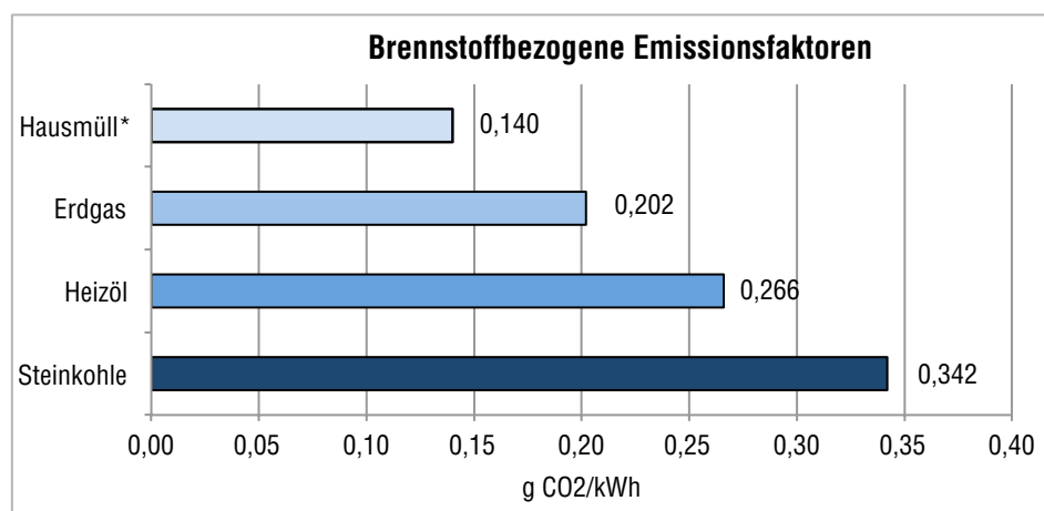
Abbildung 15: Brennstoffbezogene Emissionsfaktoren (LAK Energiebilanzen)
