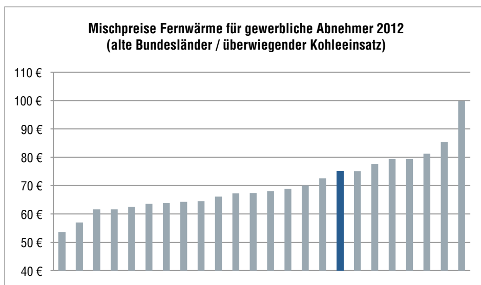
Abbildung 11: Mischpreise für gewerbliche Kunden nach Daten aus dem Fernwärmepreisvergleich 2012 des VEA e.V. für die alten Bundesländer und bei überwiegendem Kohleeinsatz (Mischpreise für eine Wärmeleistung von 600 kW und Jahresabnahmen von 900 und 1.200 MWh), dunkelblau: Vattenfall Hamburg
