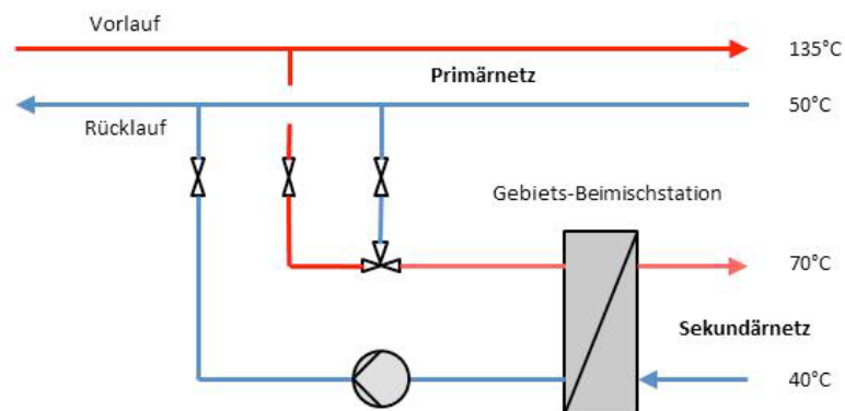
Abbildung 22: Rücklaufbeimischung mit Dreifachanschluss
