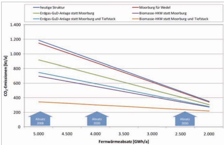
Abbildung 19: Mögliche Entwicklung der CO 2 -Emissionen der Hamburger Fernwärme (Quelle: arrhenius-Institut: Basis-Gutachten Masterplan Klimaschutz, 2011)
