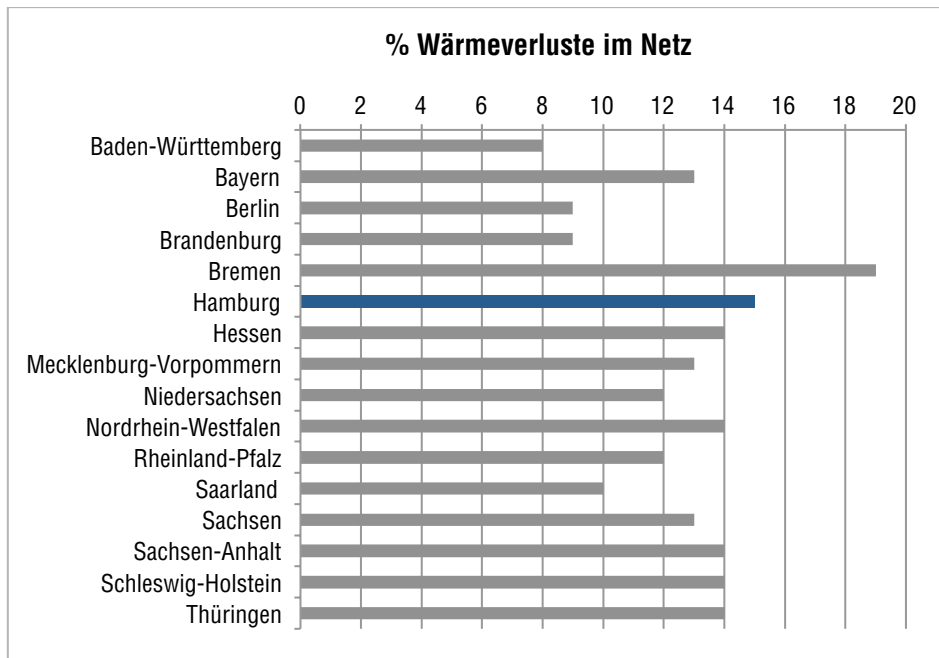
Abbildung 14: Wärmeverluste der Fernwärmenetze (Daten: AGFW Hauptbericht 2010)
