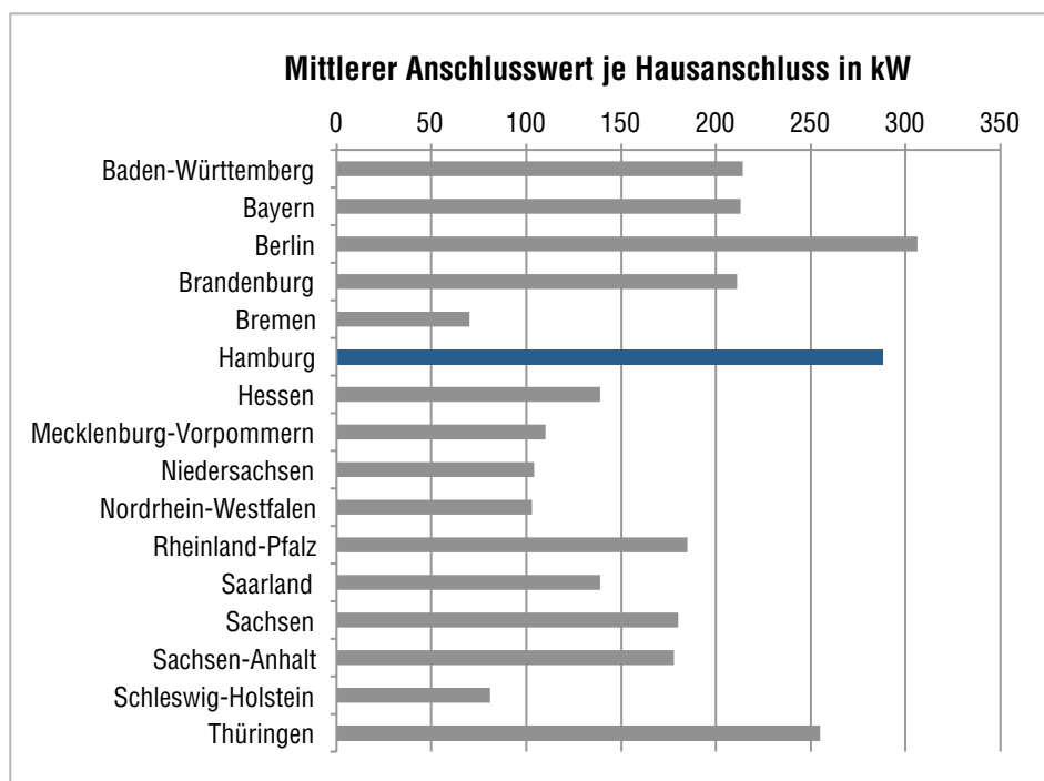
Abbildung 8: Mittlerer Anschlusswert der Hausstationen, Quelle: AGFW Hauptbericht 2010
